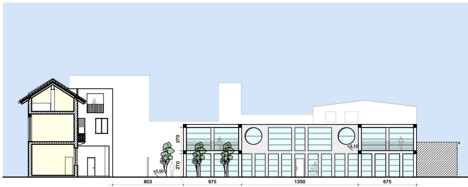
SEZIONE F - F
