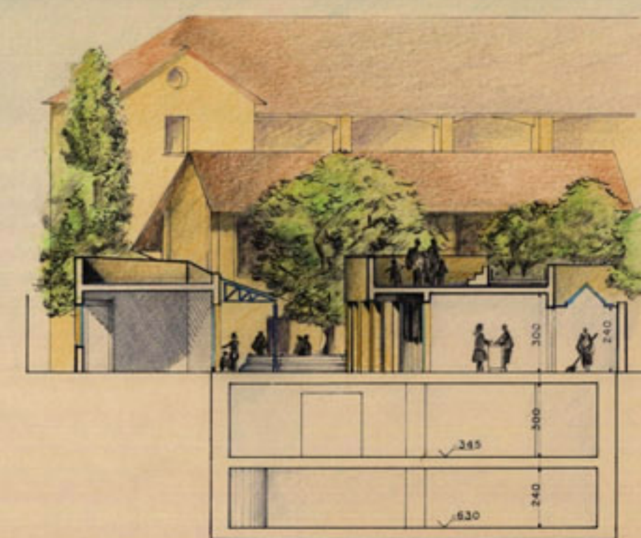
SEZIONE D-D
