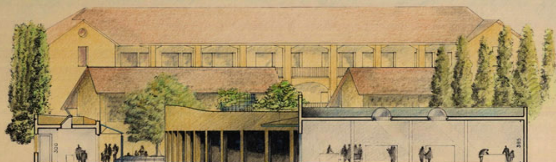
SEZIONE C-C
