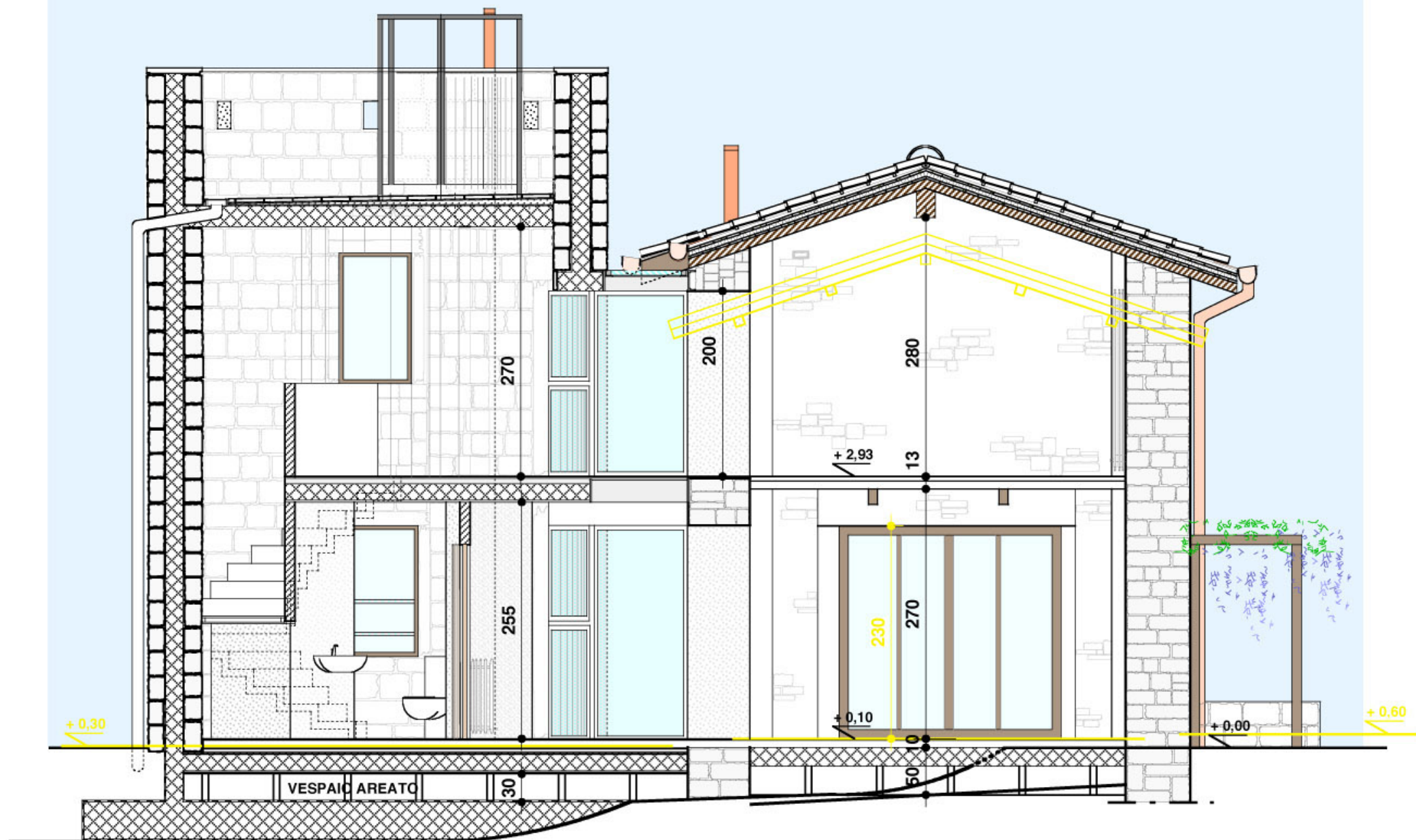
SEZIONE A-A
