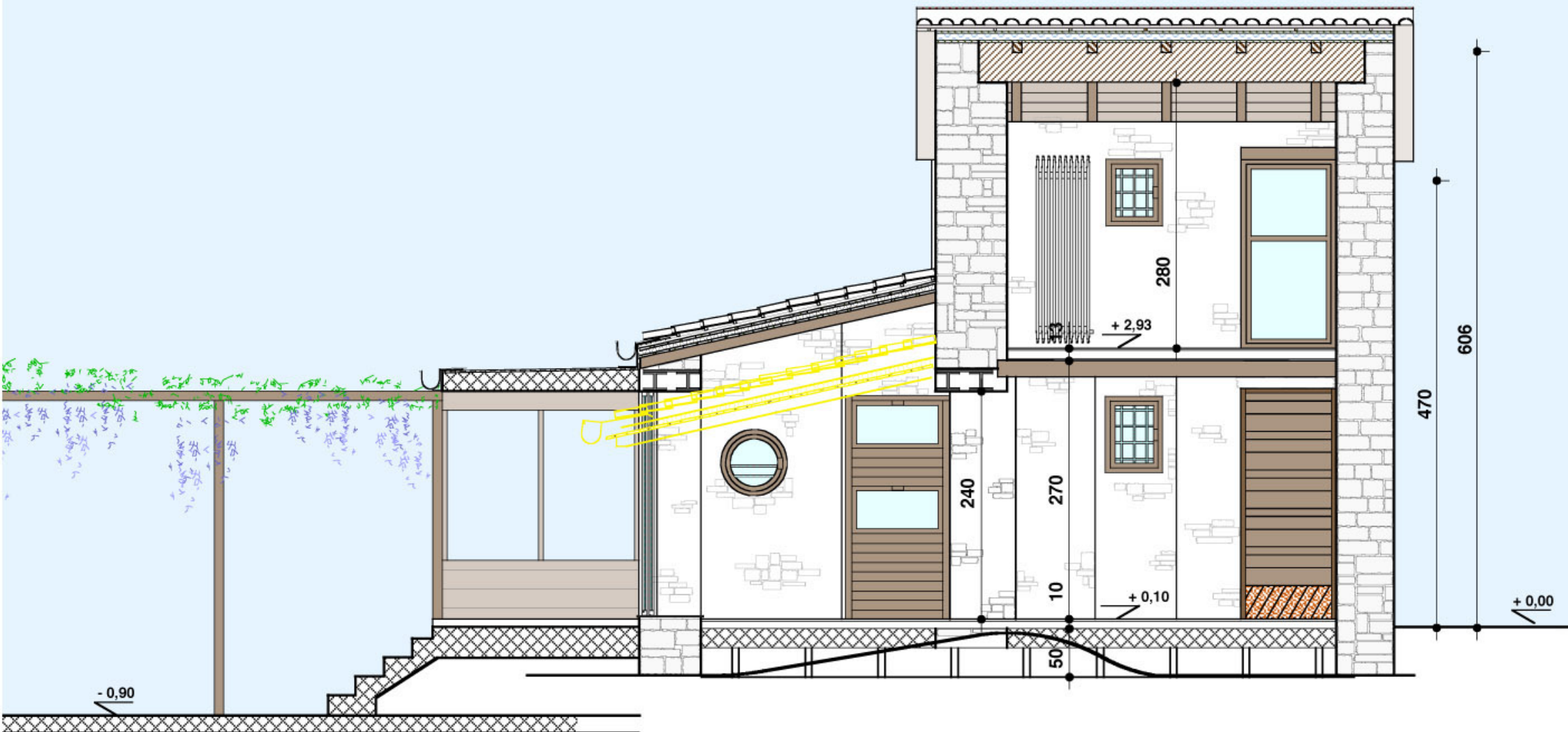
SEZIONE B-B
